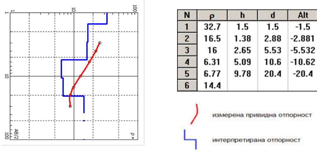
Слика 5.: Дијаграм на отпорност на сонда S3-3 Figure 5.: Diagram of resistivity on probe S3-3
